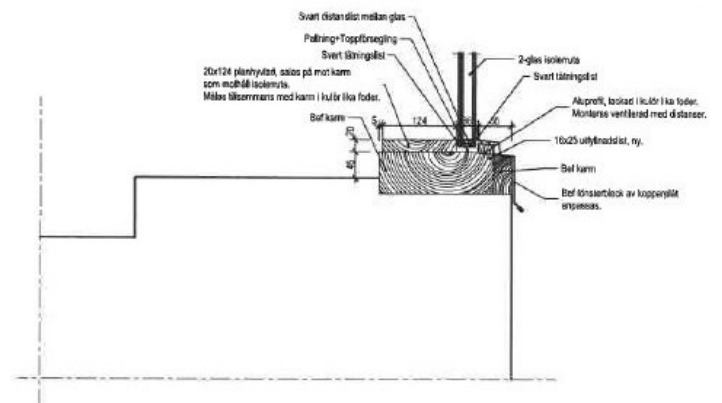
Nytt utseende. Vertikalsnitt uk.
