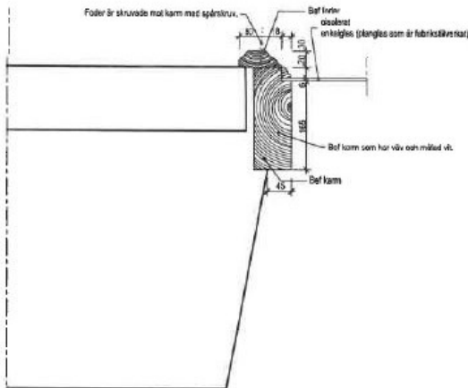
Bef utseende. horizontalsnitt sida.
