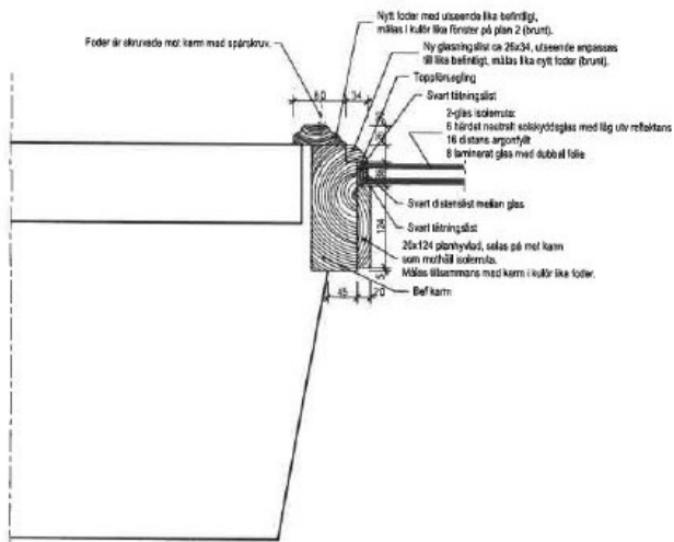
Nytt utseende. horizontalsnitt sida.
