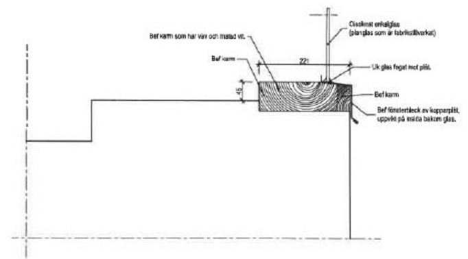
Bef utseende. Vertikalsnitt uk.
